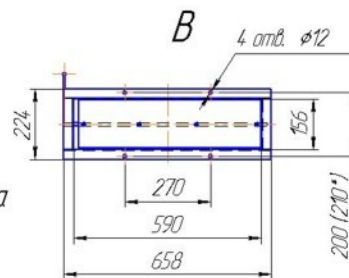
Рис. 3.1. Устройство котла. Габаритные и присоединительные размеры.
